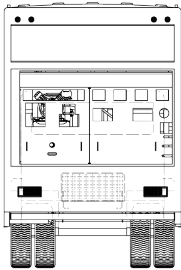
Vista trasera
